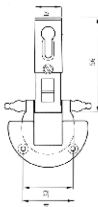
Scodellino totalmente incassato
