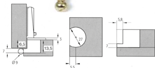
Scodellino parzialmente incassato
