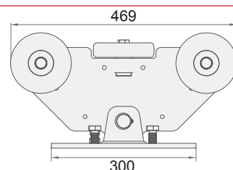
1x CG-21G
