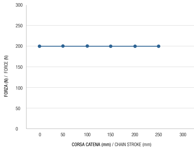
L20 Insert - Portate attuatori vasistas L20 Insert - Actuator force - bottom hung
