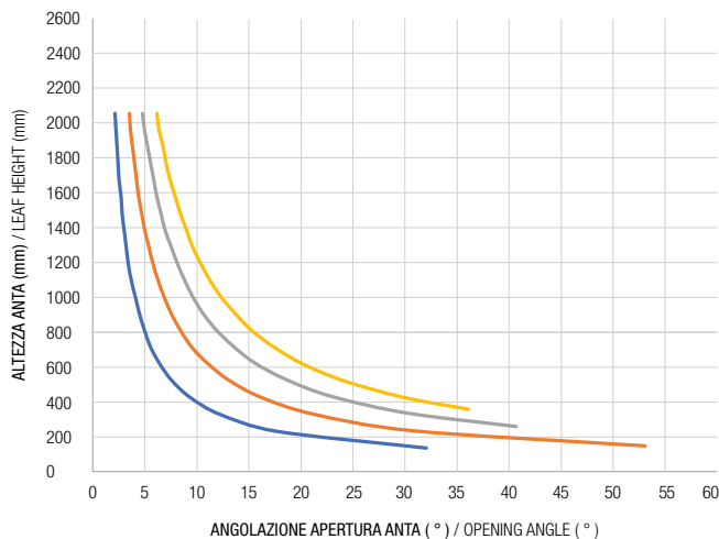
L20 Insert - Angolo di apertura anta vasistas L20 Insert - Bottom hung opening angle
